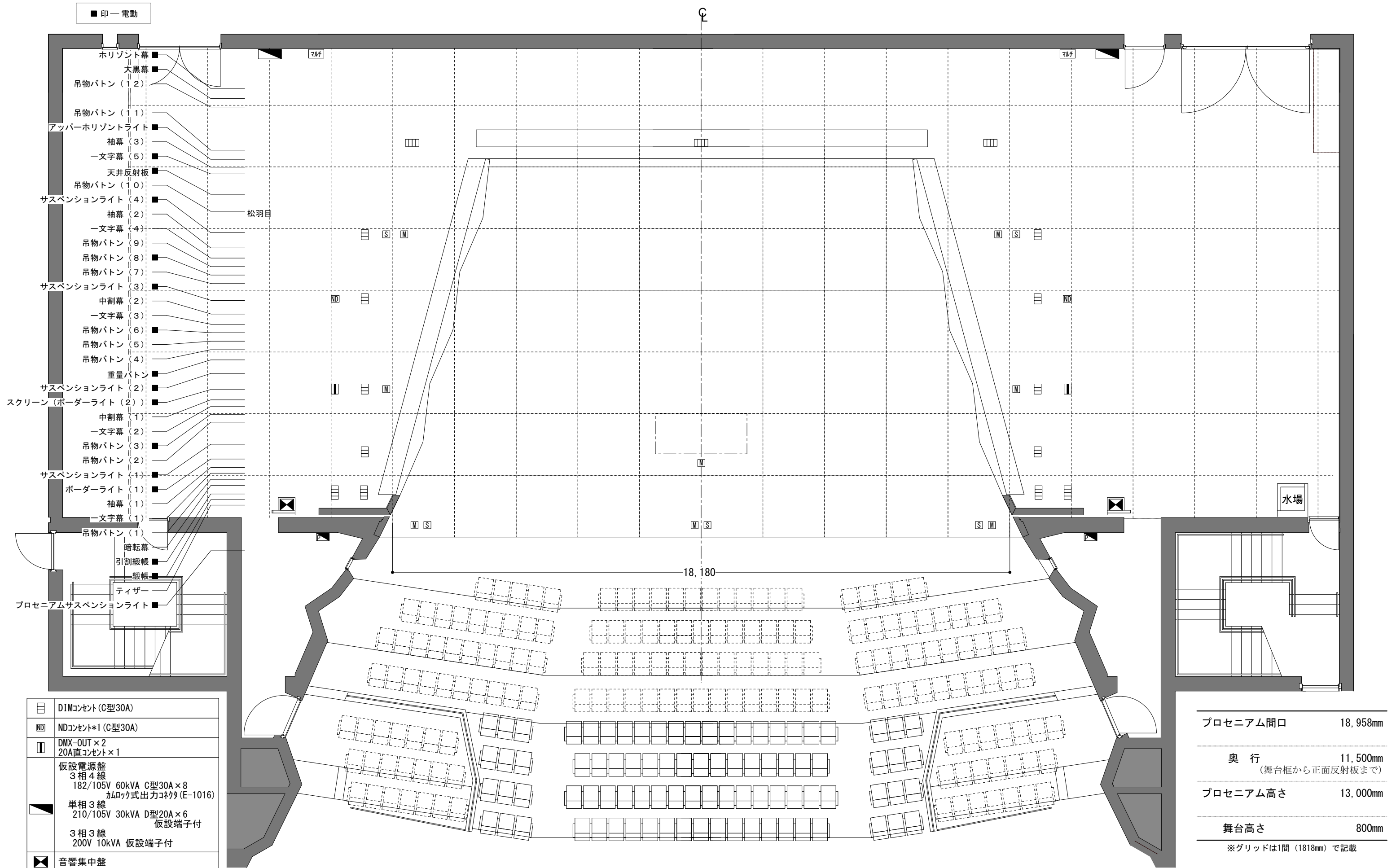
舞台平面図 S = 1 : 100 (A3印刷の場合)
